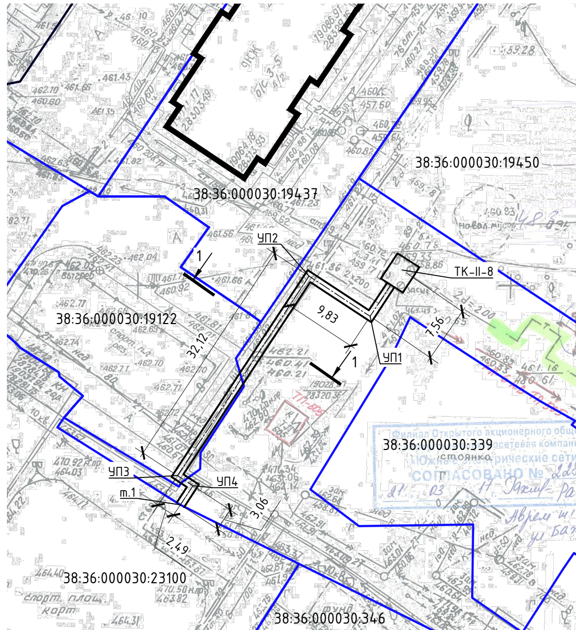
План тепловой сети
